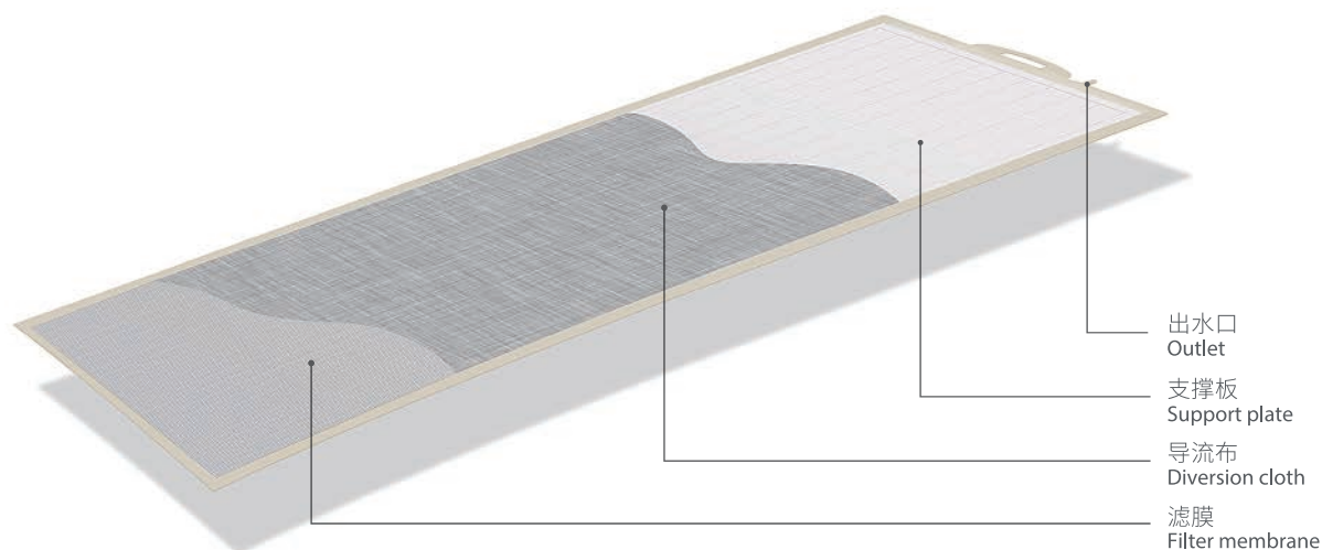
平板膜元件构造图 Flat-sheet membrane unit structure diagram
